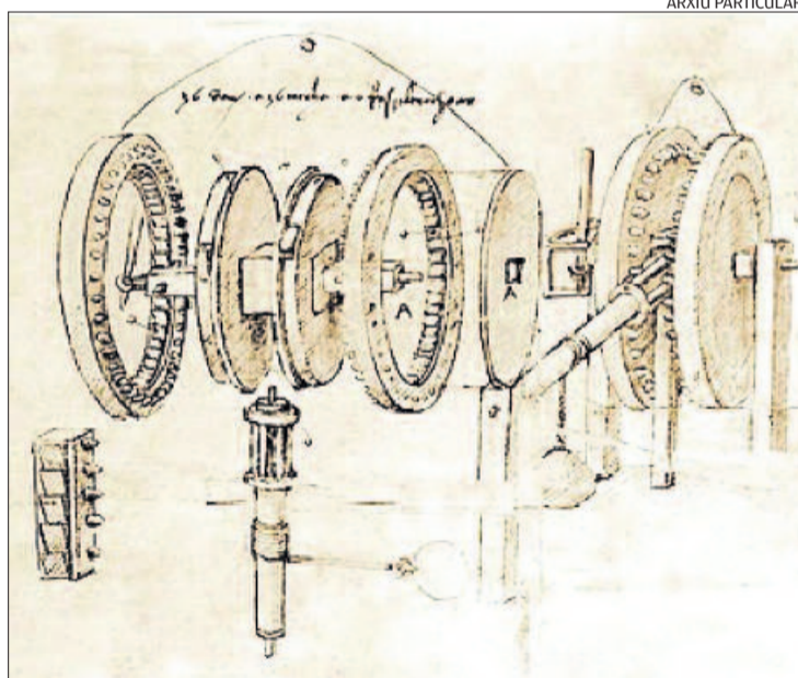
Imatge del llibre de Romano Nanni «Leonardo e le arti meccaniche»
